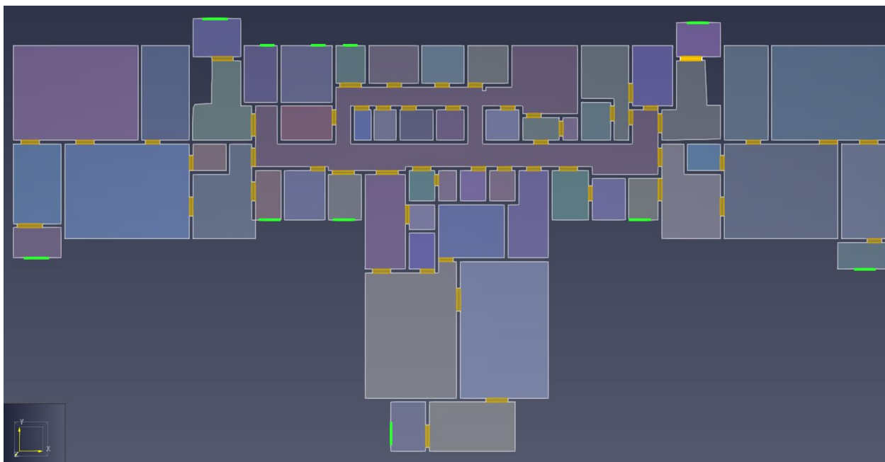
Рисунок 1 – Отрисовка комнат, дверей и эвакуационных выходов.
