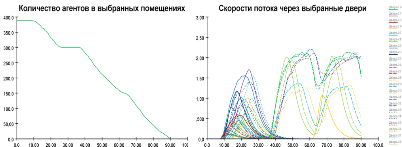
Рисунок 4 – Построение графиков.
