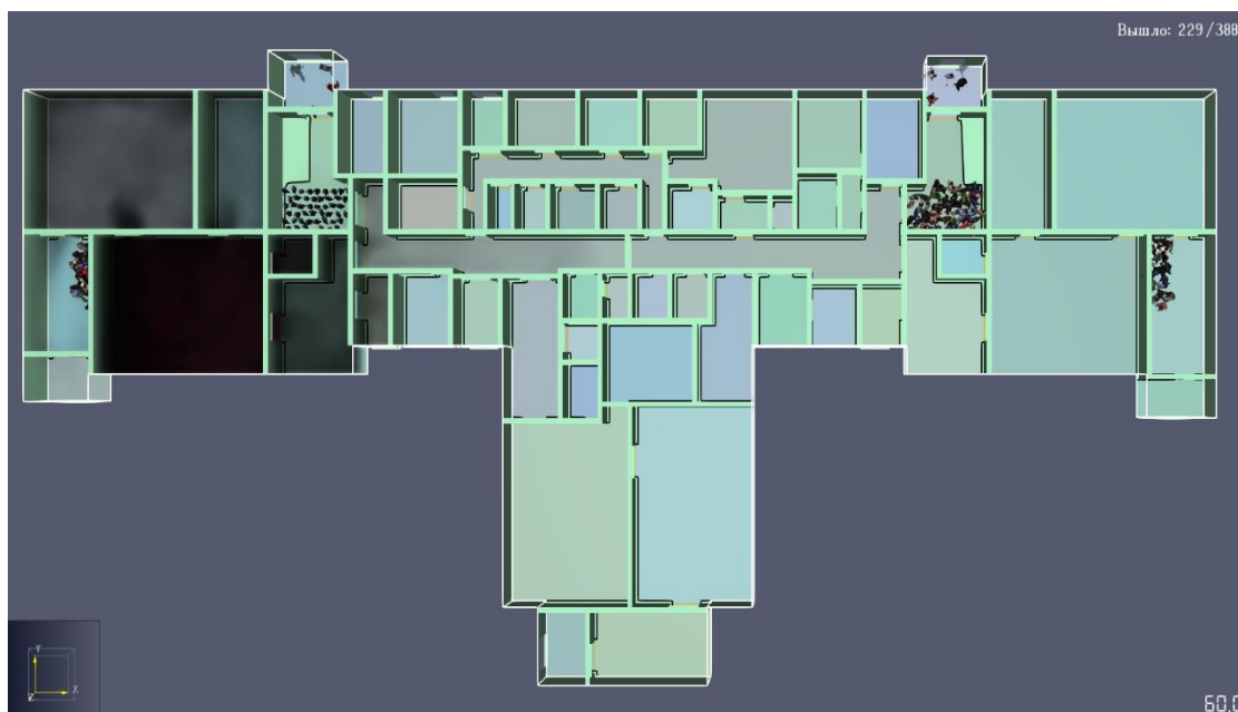
Рисунок 3 – Моделирование процесса эвакуации.
